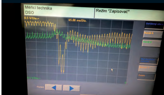
➔ Naměřený záznam v okamžiku projevu závady. Žlutá křivka – signál snímače množství nasávaného vzduchu, zelená křivka – signál snímače plnicího tlaku.
